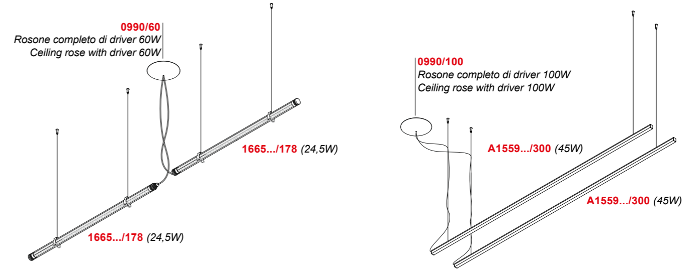
Kit di fissaggio a sospensione fornito con la lampada - Suspension fixing kit supplied with the lamp
